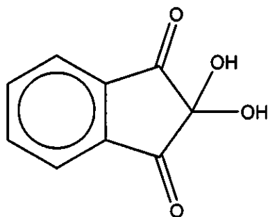
ninhydrin
