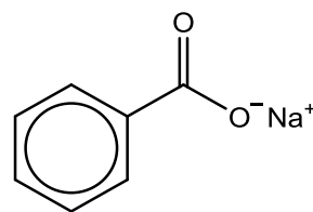
sodium benzoate
