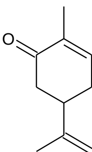
Carvone
