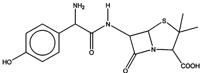
Amoxicillin
