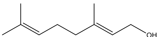
Geraniol
