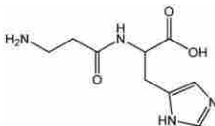
carnosine
