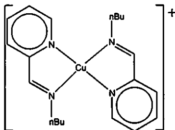
Cu(I)-nBuPCA catalyst
