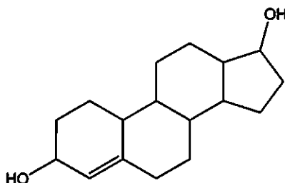
Bolandiol
