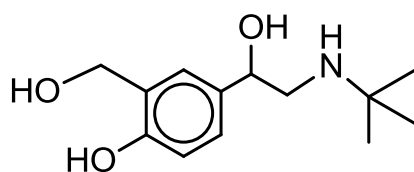
salbutamol
