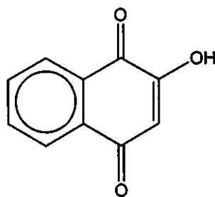
Lawsone
